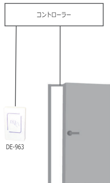
機器系統図
